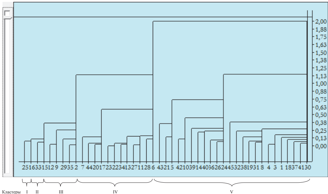
Рис. 6. Дендрограмма кластеризации по максимуму коэффициента корреляции между сортообразцами в коллекционном питомнике овса ярового 2010 г. посева
