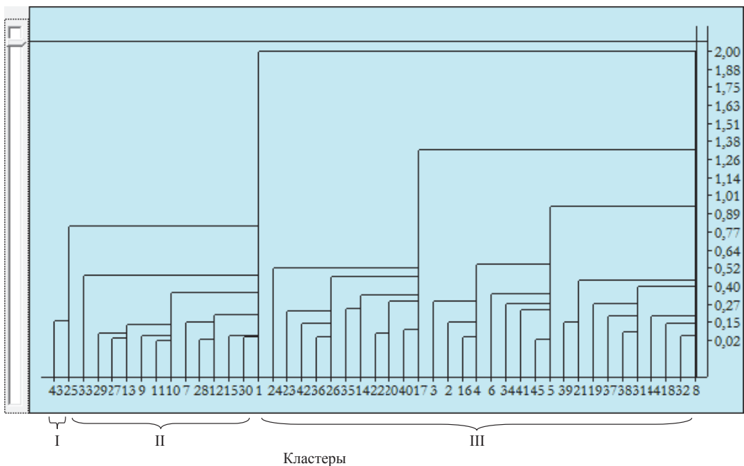
Рис. 5. Дендрограмма кластеризации по максимуму коэффициента корреляции между сортообразцами в коллекционном питомнике овса ярового 2009 г.
