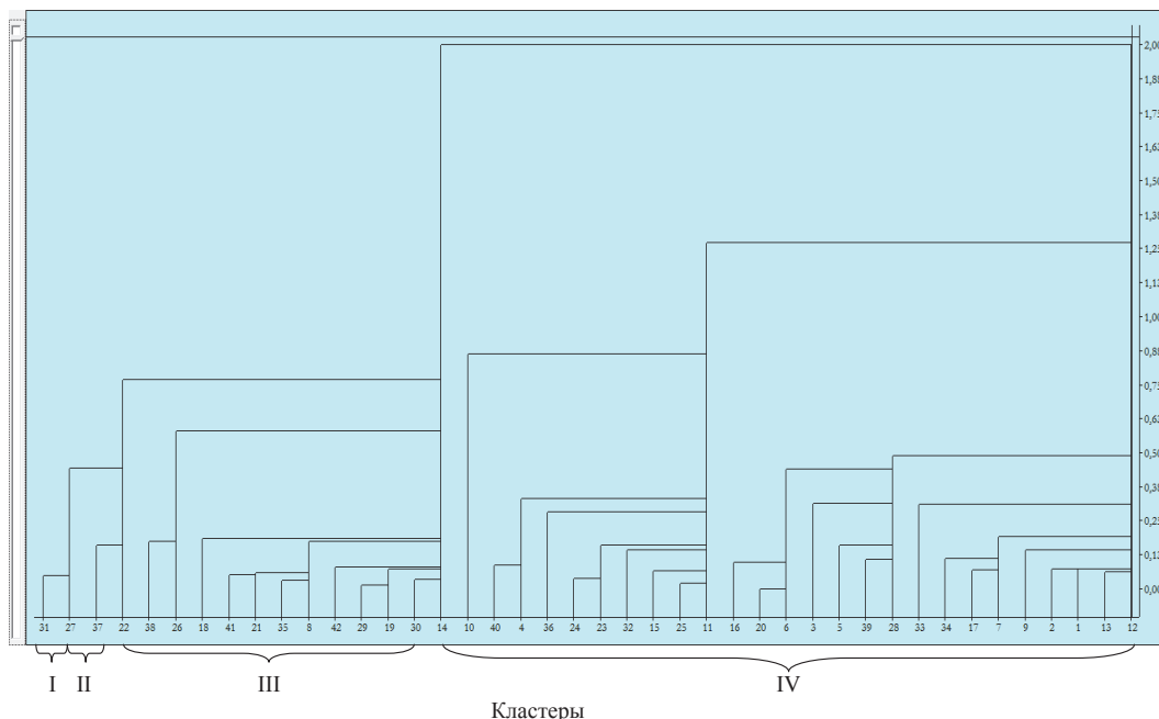
Рис. 4. Дендрограмма кластеризации по максимуму коэффициента корреляции между сортообразцами в коллекционном питомнике овса ярового 2008 г. (расшифровка номеров представлена в табл. 1)
