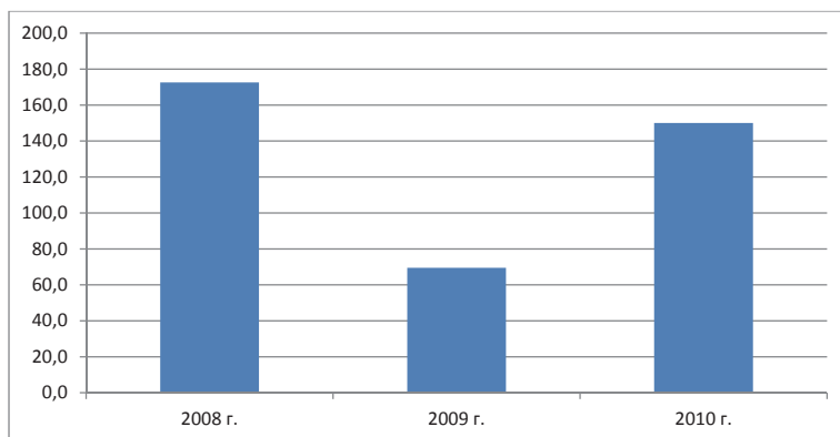
Рис. 2. Сумма осадков при температуре воздуха выше 10°C, мм
