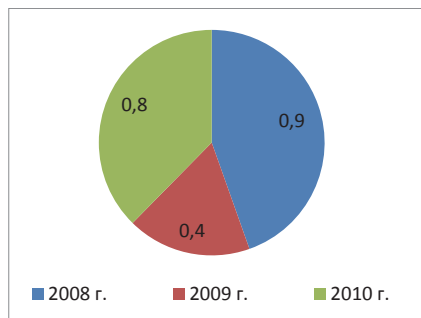
Рис. 3. Значение Гидротермического коэффициента (ГТК) в вегетационный период 2008–2010 гг.
