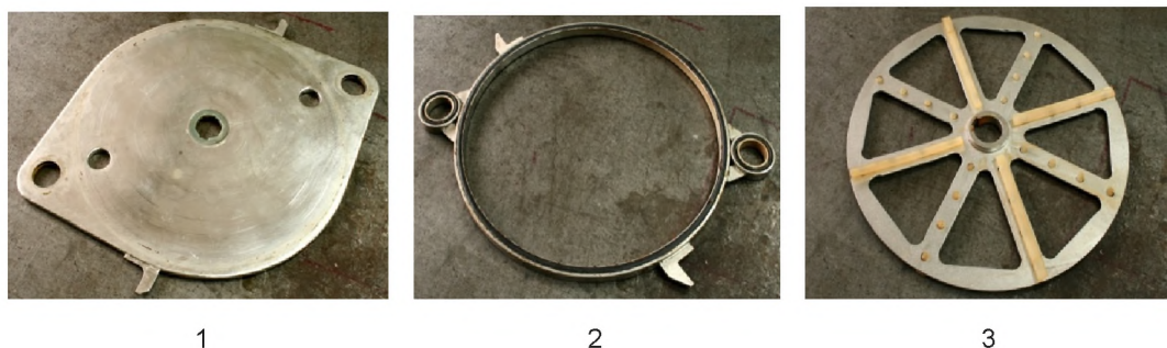
Рис. 1. Элементы пластинчатого скребкового теплообменника: 1 — продуктовая пластина; 2 — уплотнительное кольцо; 3 — скребок-мешалка
