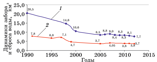
Динамика забора воды на орошение и сброса дренажного стока (по данным Государственных докладов «О состоянии и об охране окружающей среды Российской Федерации»)
