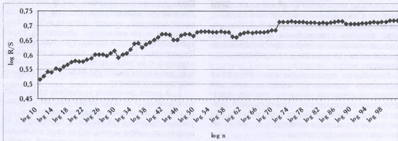
Рис. 1. R/S-анализ урожайности зерновых культур по России/СССР/России за период 1801-2003 гг.
