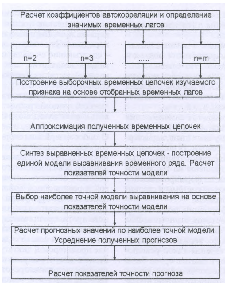
Рис. 2. Алгоритм построения прогноза урожайности зерновых культур на основе выборочных временных цепочек
