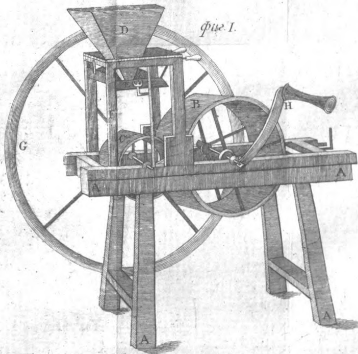
Машина для раздавливанія солода
