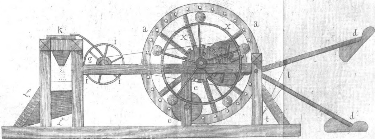
Машина для раздавливанія солода
