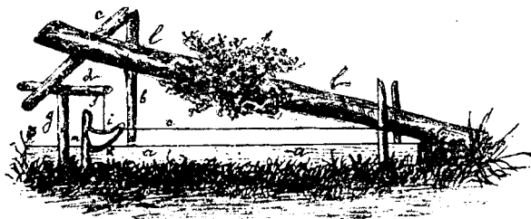
Рис. 22. Поѣдная пасть.
