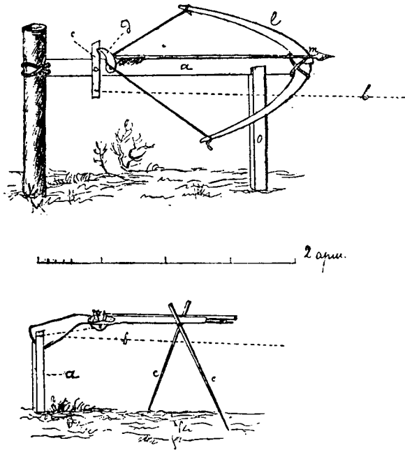
Рис. 39. Настороженные самострѣлъ и винтовка.
