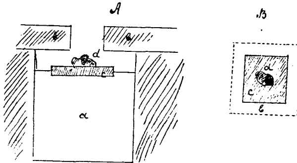
Рис. 48. Яма изъ льдинъ для ловли песцовъ. А.—Вертикальный разрѣзъ. В.—Видъ сверху.
