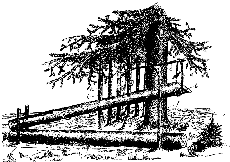
Рис. 24. Кряжъ на зайца.
