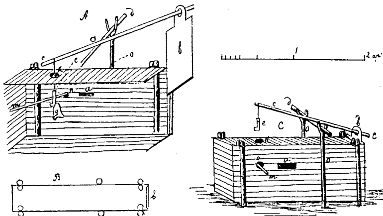
Рис. 50. Кулёма на лисицу. А. Настороженная ловушка въ разрѣзѣ. В. Горизонтальная проекція. С. Общій видъ захлопнувшейся ловушки.
