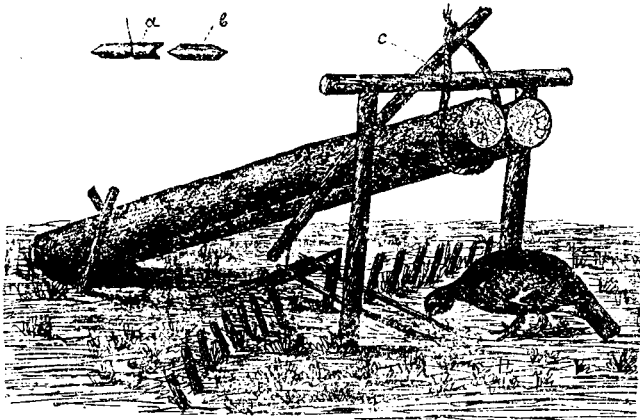
Рис. 18. Слопецъ на глухаря.
