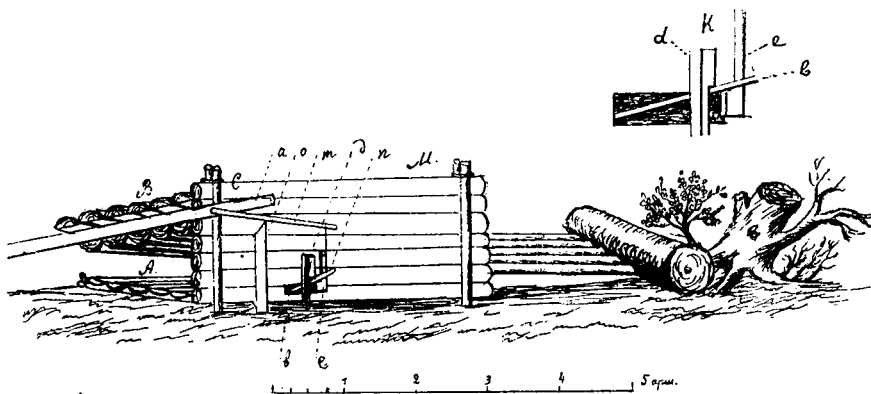
Рис. 20. Пастъ на лисицу.
