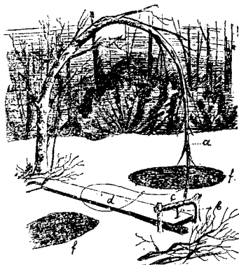
Рис. 15. Пружокъ на глухаря.
