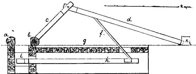
Рис. 35. Жомъ.
