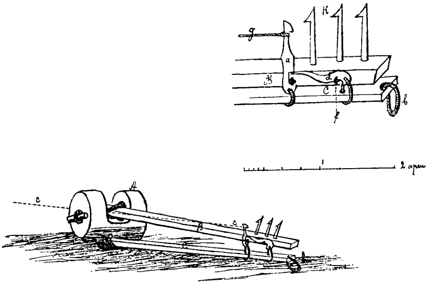
Рис. 41. Кляпцы.
