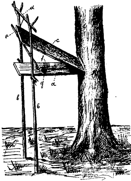
Рис. 27. Плашка для куницъ.
