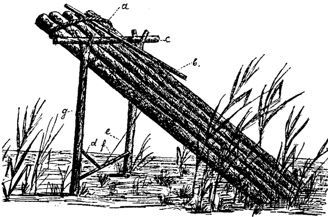
Рис. 17. Слопецъ на зайца.
