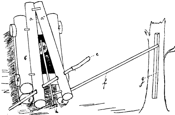
Рис. 34. Щемиха. Планъ устройства.
