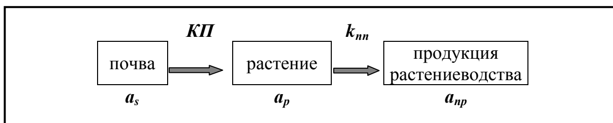
Рис. 1. – Схема миграции радионуклида в продукцию растениеводства
