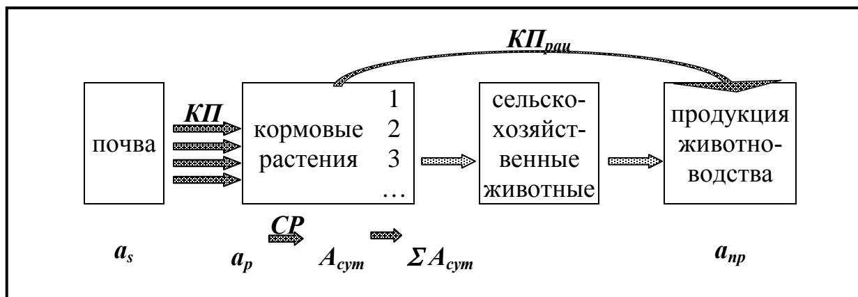
Рис. 2. Схема миграции радионуклида в продукцию животноводства
