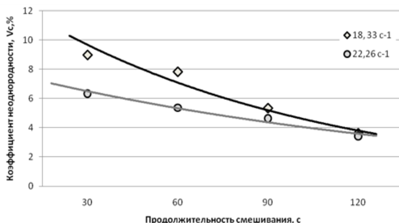
Рисунок 3.4 - Кривая кинетики процесса смешивания
