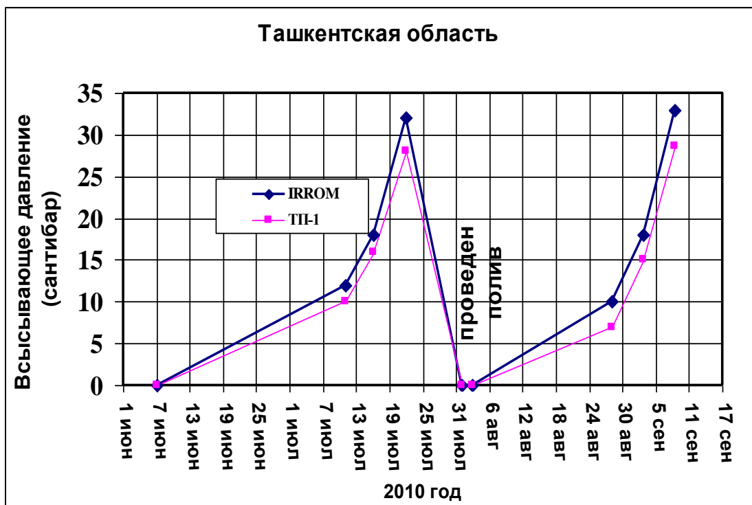
Рис. 3.5. Динамика всасывающего давления почв по показаниям тензиометров ТП-1 и IRROMETER (Ташкентская область)
