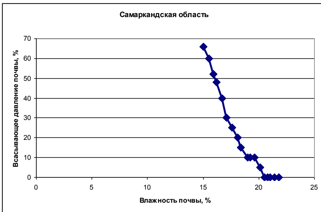
Рис. 3.13. Зависимость всасывающего давления от влажности почвы в период между вторым и третьим поливом
