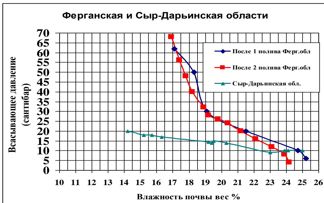
Рис. 3.7. Зависимость всасывающего давления тензиометров ТП-1 от влажности почвы (Ферганская и Сырдарьинская области)
