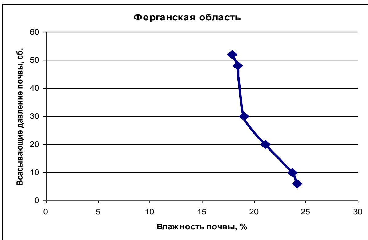
Рис. 3.8. Зависимость всасывающего давления от влажности почвы в период между первым и вторым поливом
