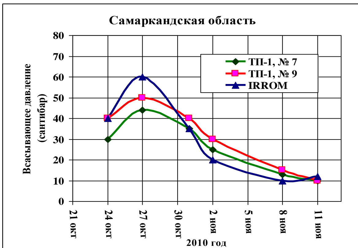
Рис. 3.6. Динамика всасывающего давления почв по показаниям различных тензиометров (Самаркандская область)
