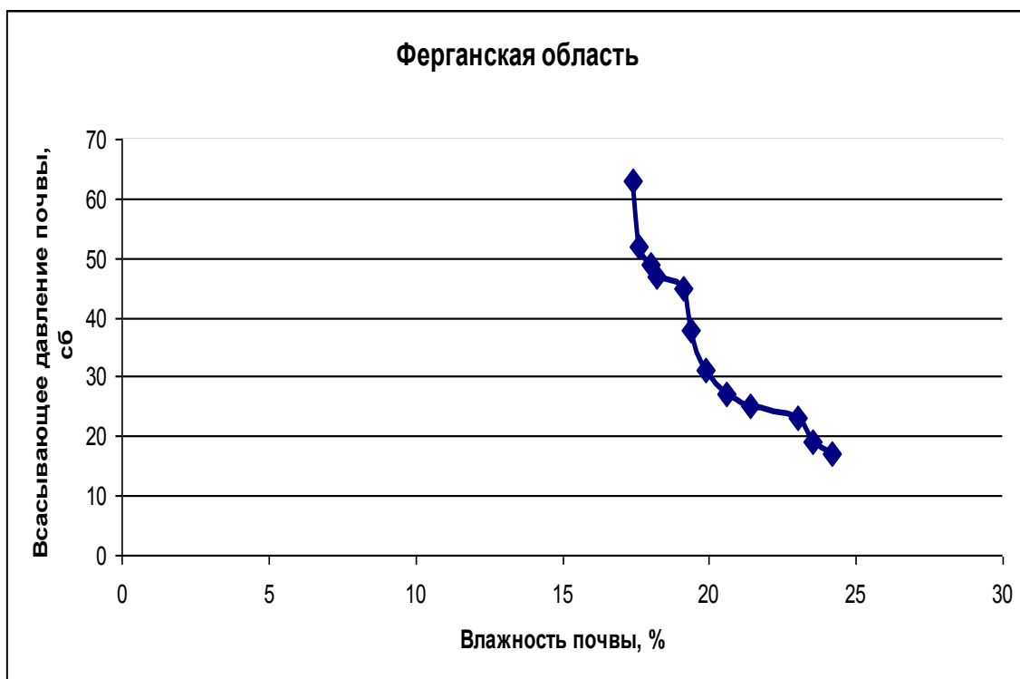
Рис. 3.9. Зависимость всасывающего давления от влажности почвы в период между вторым и третьим поливом
