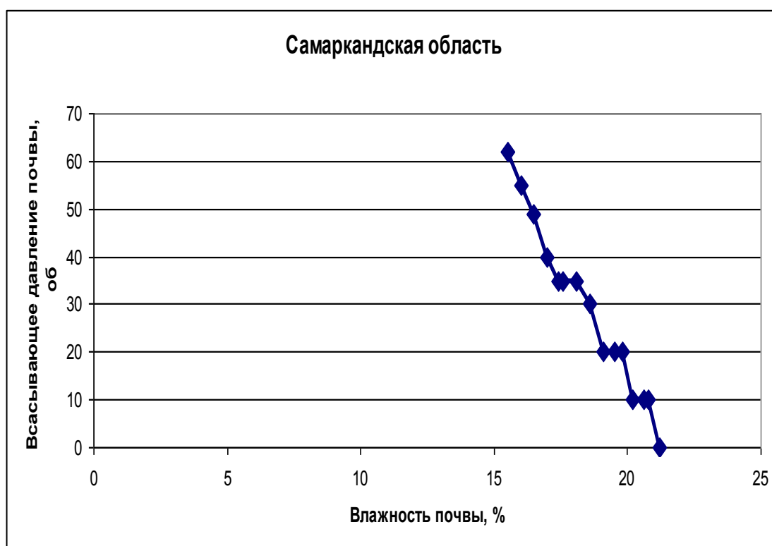
Рис. 3.11. Зависимость всасывающего давления от влажности почвы в период до первого полива
