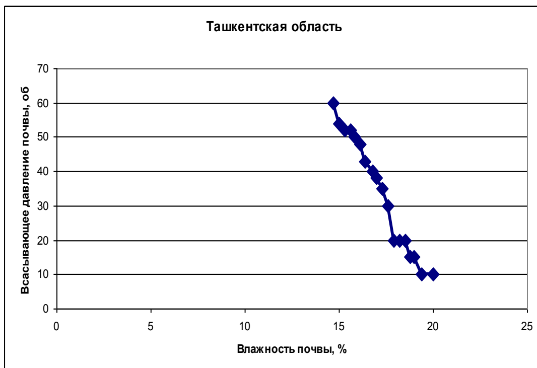
Рис. 3.16. Зависимость всасывающего давления от влажности почвы в период между третьим и четвертым поливом
