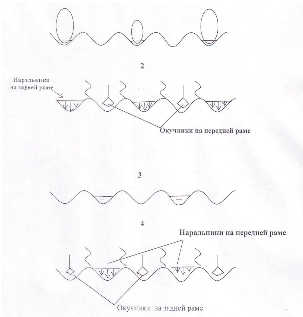
Рис. 8.1. Расположение рабочих органов тракторного культиватора при поливе хлопчатника по чередующимся бороздам (ширина междурядий 60 см: 1. Полив по следу задних колес трактора; 2. Расположение рабочих органов тракторного культиватора после полива; 3. Полив по межколесным бороздам; 4. Расположение рабочих органов тракторного культиватора после полива по межколесным бороздам
