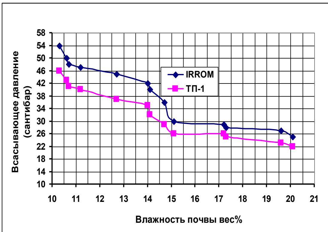
Рис. 3.4. Зависимость всасывающего давления от влажности почвы
