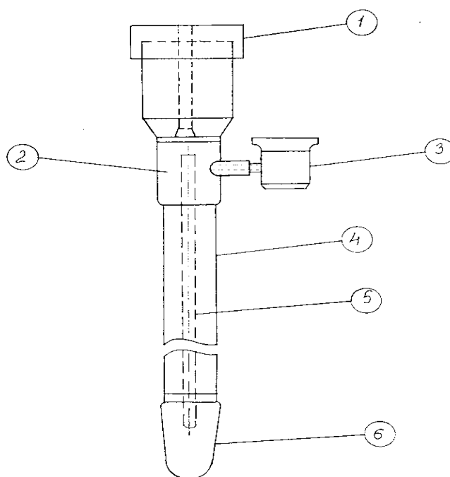
Рис. 3.1. Конструкция тензиометра «Иррометр», где: 1-крышка с пробкой; 2-воздухоулавливатель; 3-вакуумметр; 4-защитный корпус из прозрачного оргстекла; 5-трубка, заполняемая химически чистой водой; 6-керамический наконечник (фильтр)
