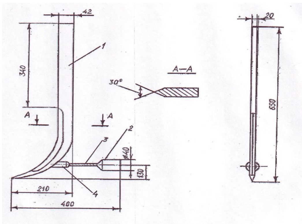
Рис. 7.1. Рабочий орган для устройства кротовин: 1 – нож-щелерез, 2 – кротователь, 3 – тяговый трос, 4 - хвостовик
