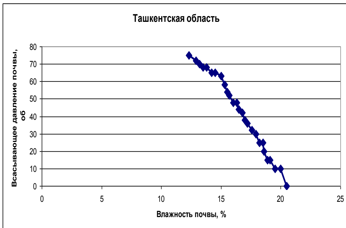
Рис. 3.17. Зависимость всасывающего давления от влажности почвы в период между четвертым и пятым поливом
