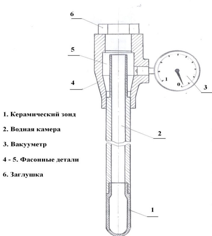
Рис. 3.3. Конструкция тензиометра ТП-1
