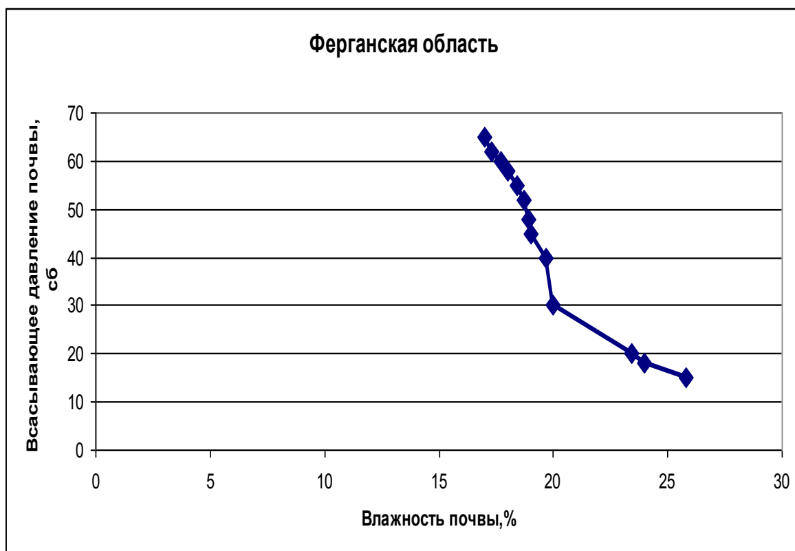
Рис. 3.10. Зависимость всасывающего давления от влажности почвы в период между третьим и четвертым поливом
