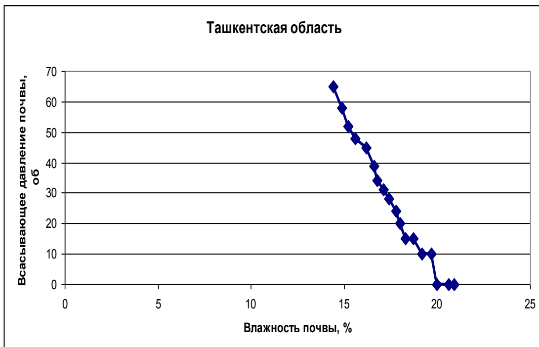
Рис. 3.15. Зависимость всасывающего давления от влажности почвы в период между вторым и третьим поливом
