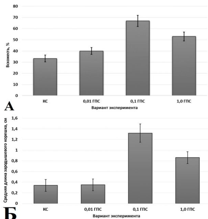
Рис. 1 Всхожесть и прораствание семян тест-культуры в условиях смоделированного солевого стресса
