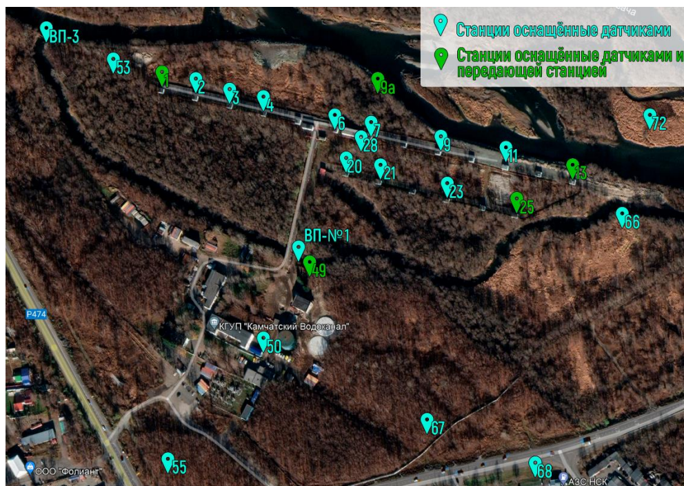
Рис. 1 Автоматизированная система контроля показателей подземных вод скважинного водозабора «Авачинский».
