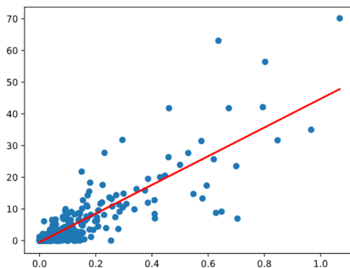
Рис. 4 Диаграмма рассеяния
