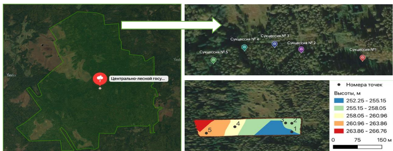
Рис. 1 Расположение ключевых участков в урочище Красное
