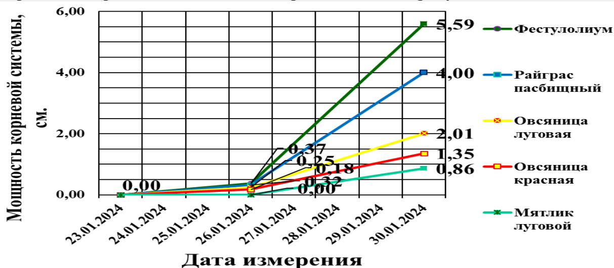
Рис. 3 Мощность корневой системы, см.
