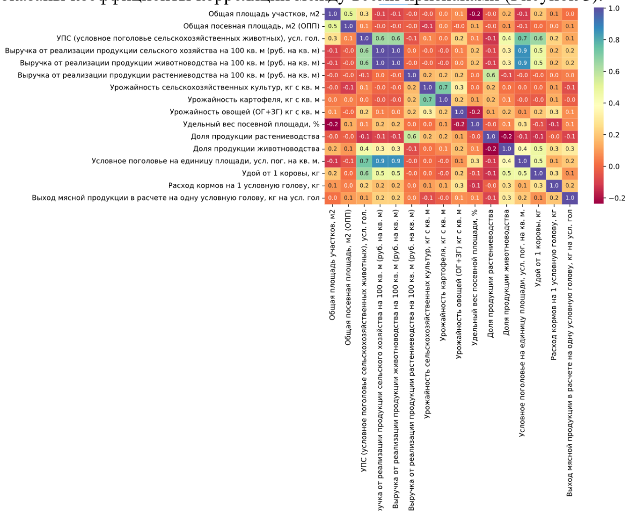
Рис. 10 Тепловая карта
