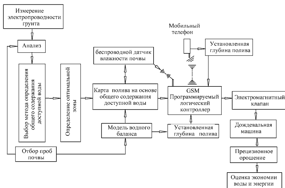
Рис. 2. Стратегия точного орошения
