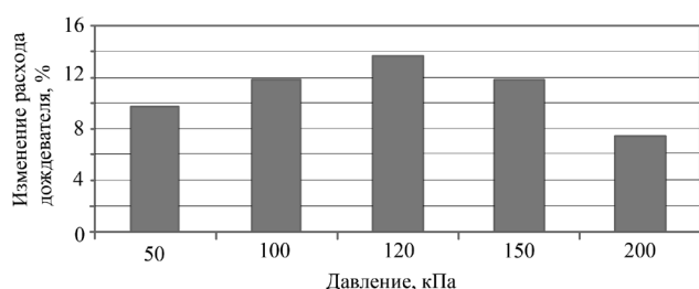
Рис. 5. Зависимость между рабочим давлением и изменением расхода дождевателя
