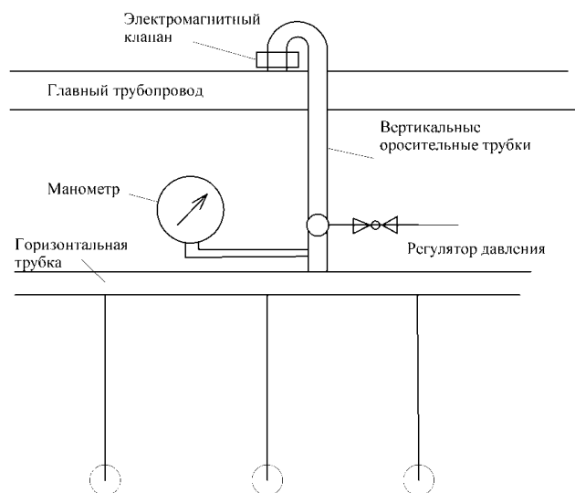
Рис. 3. Вариант с блочным управлением дождевателями по ускоренной схеме
