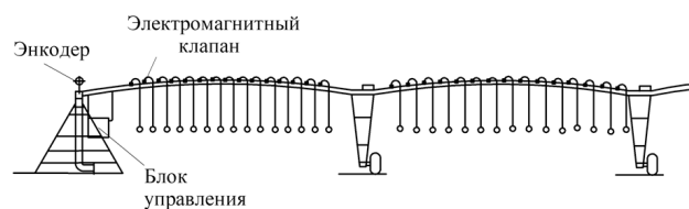
Рис. 1. Модернизация дождевальной машины
