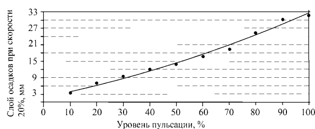
Рис. 6. Изменение слоя осадков в зависимости от режима полива
