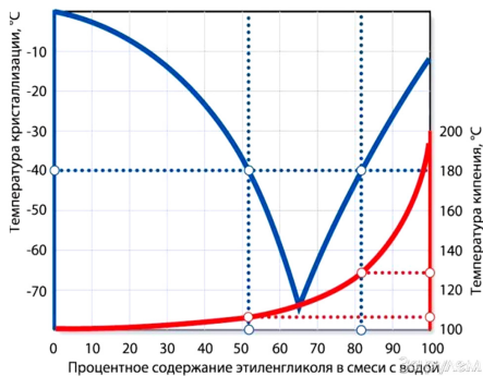
Рис. 38. Кривая кристаллизации водноэтиленгликолевых смесей.
