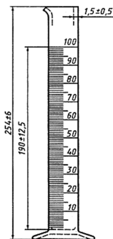
Рис. 14. Мерный цилиндр ёмкостью 100 см 3 , с ценой деления 1 см 3
