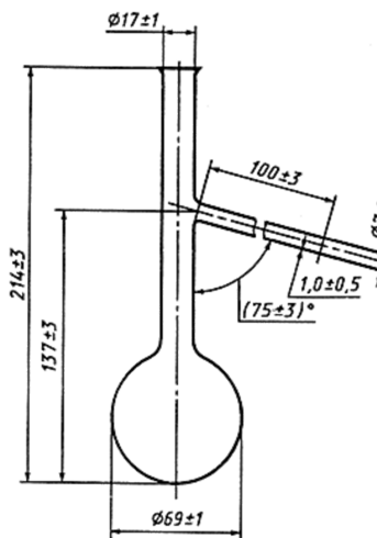
Рис. 13 Колба для перегонки КРН-125
