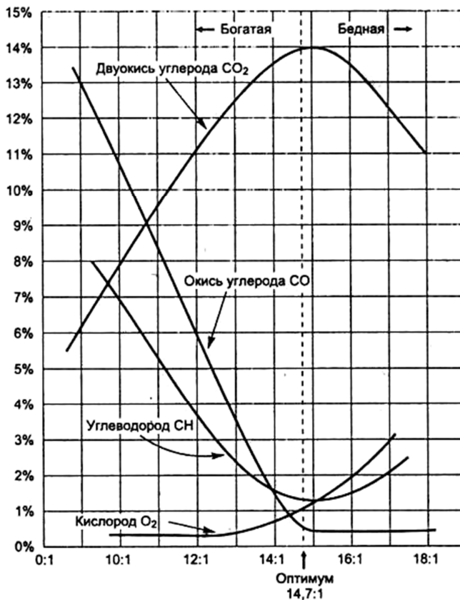
Рис. 6. Содержания CH, CO, O 2 , CO 2 в выхлопных газах от соотношения воздух /топливо в смеси.
