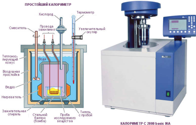
Рис.1. Калориметрическая установка
