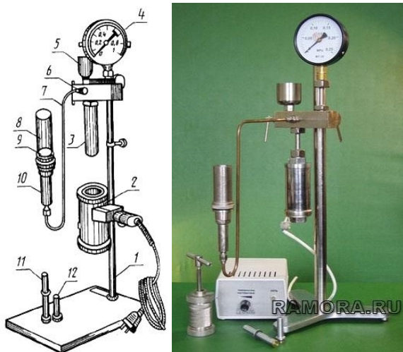
Рис. 33. Пластометр К-2:
