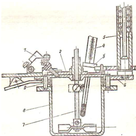
Рис. 26. Аппарат для определения температуры вспышки:
