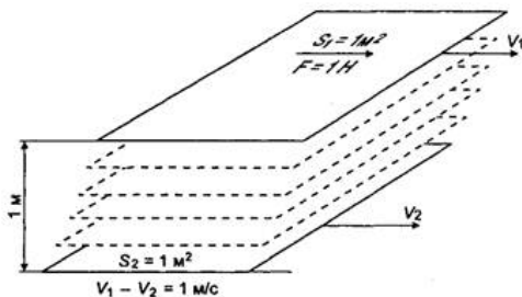
Рис. 28. Схема взаимного перемещения слоев жидкости.
