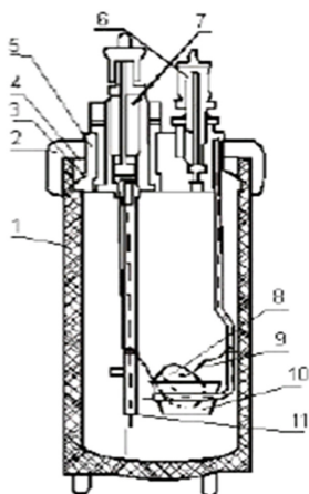
Рис.2. Калориметрическая бомба:
