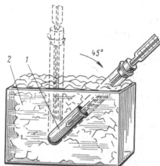
Рис. 21. Схема прибора для определения температуры застывания дизельного топлива:
