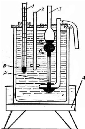
Рис. 30. Прибор для определения кинематической вязкости нефтепродукта:
