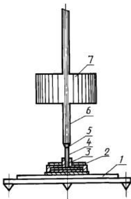
Рис. 35. Схема прибора КСА для определения коллоидной стабильности: 1 – кронштейн; 2 – стальная шайба; 3 – чашечка; 4 – поршень; 5 – шарик; 6 – шток; 7 – груз.
