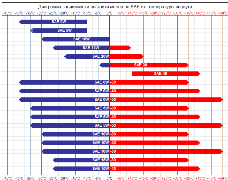
Рис.32. Диаграмма зависимости вязкости масла по SAE от температуры воздуха.
