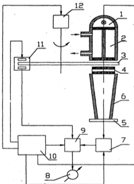
Рис. 4. Блок-схема газоанализатора:
