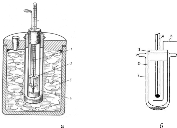
Рис. 22. Схема прибора для определения температуры помутнения дизельного топлива: а) 1 - мешалка; 2 - испытуемое топливо; 3 - охлаждающая смесь; 4 - воздух; б) 1 — пробирка наружная; 2 — пробирка внутренняя; 3 — пробка; 4 — термометр; 5 — мешалка
