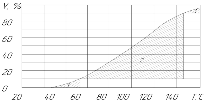
Рис. 7. Кривая разгонки автомобильного бензина, фракции: 1 - пусковая, 2 - рабочая, 3 - концевая .
