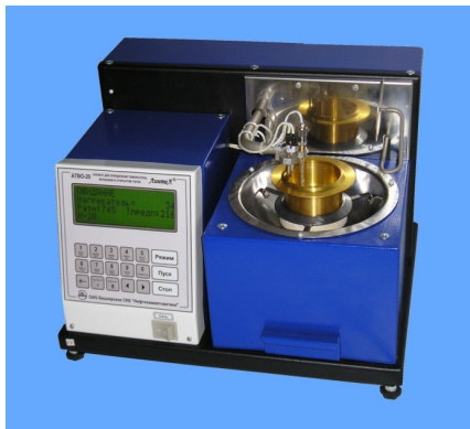
Рис. 25. Автоматический аппарат для определения температуры вспышки АТВ-20
