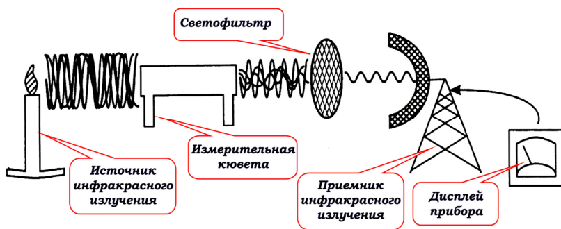
Рис. 3. Схема работы автомобильного газоанализатора
