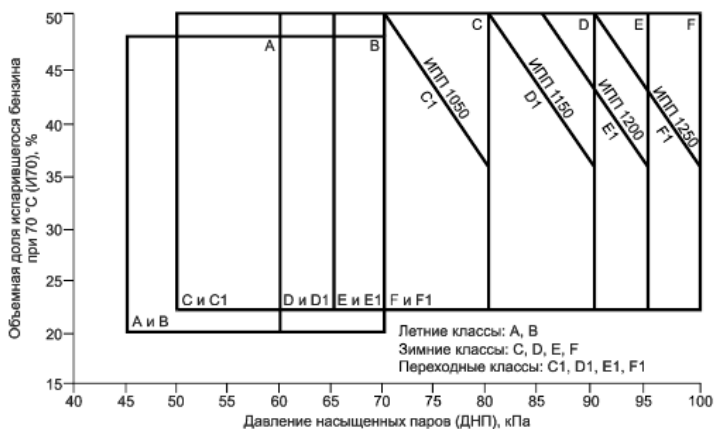
Рис. 17. Диаграмма определения классов испаряемости бензинов
