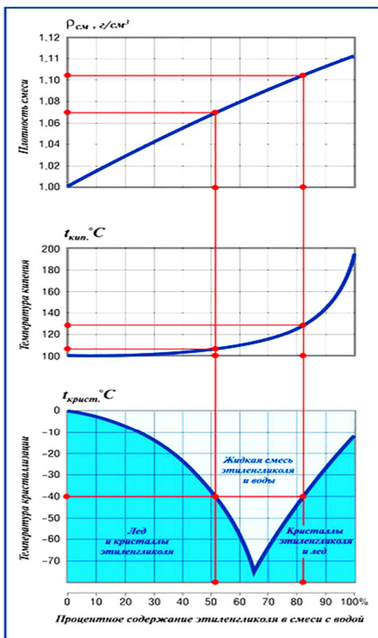
Рис. 39. Температура кристаллизации, температура кипения, плотность смеси этиленгликоля и воды в зависимости от содержания в ней этиленгликоля
